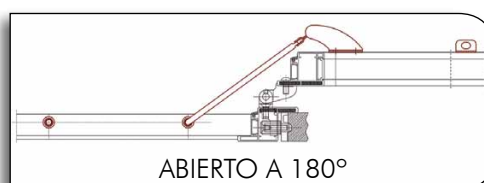
Ref: RETE200 (Para hojas menores de 450 mm.) Ref: RETE300 (Para hojas mayores de 450 mm.)
